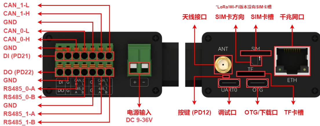
ECM31-B 接口功能图
